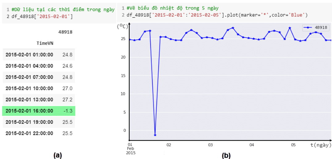
Hình 11. Kiểm chứng điểm ngoại lai trái có giá trị thấp nhất tại trạm 48918.
