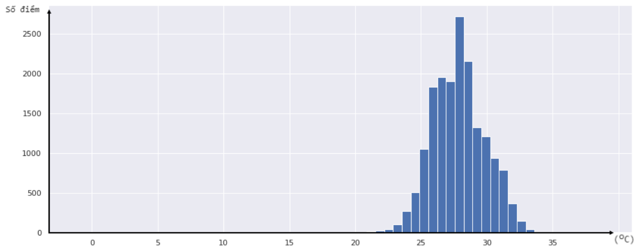
Hình 7. Biểu đồ histogram của tập dữ liệu nhiệt độ trạm 48918.
