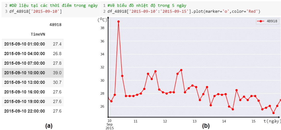
Hình 12. Kiểm chứng điểm ngoại lai phải có giá trị cao nhất tại trạm 48918.
