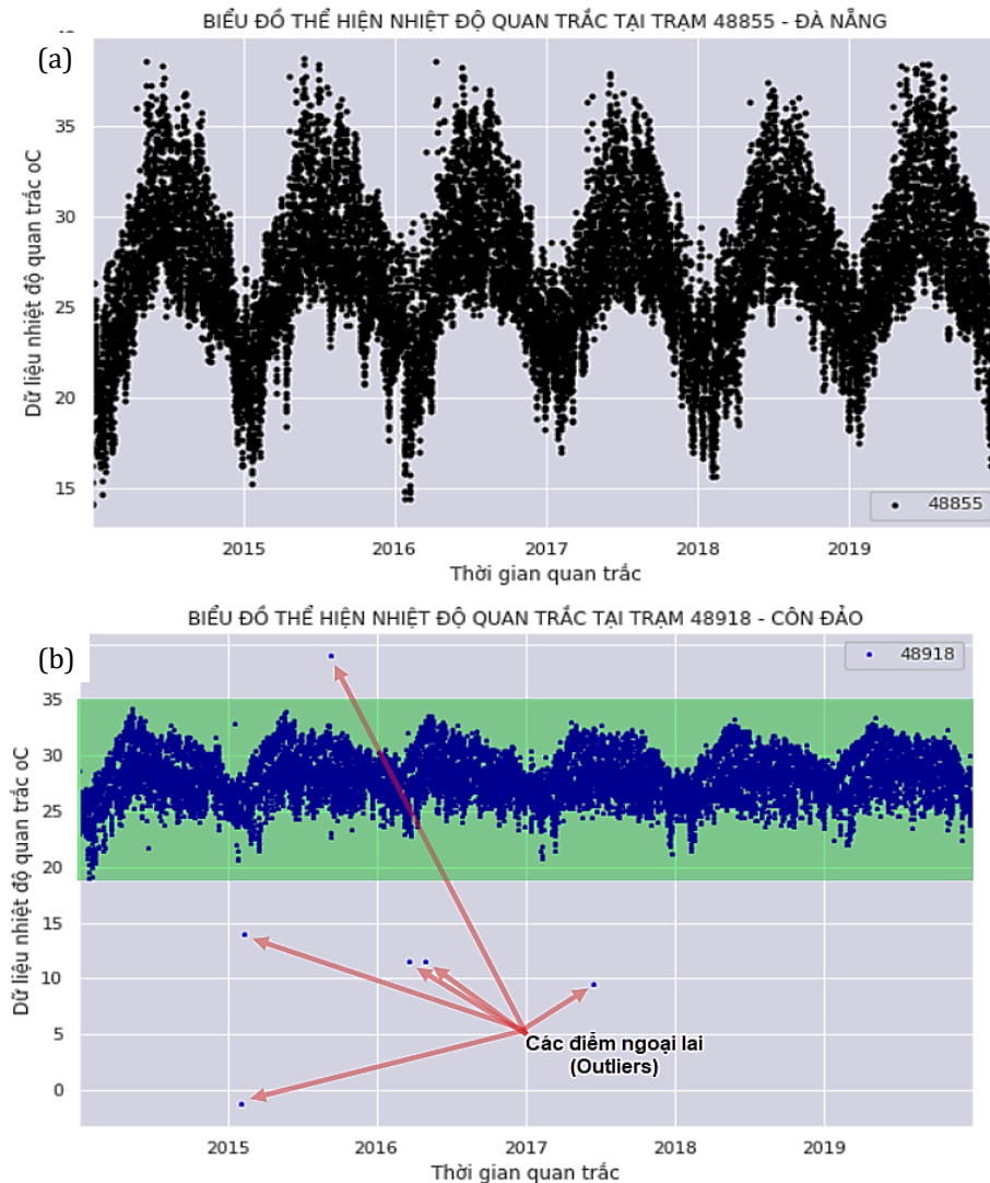
Hình 3. (a) Minh họa tập dữ liệu không chứa dữ liệu ngoại lai; (b) Minh họa tập dữ liệu chứa các điểm dữ liệu ngoại lai.
